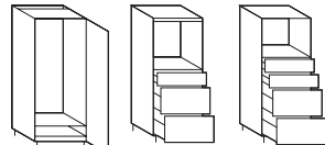
1 door width 45, 60 cm
